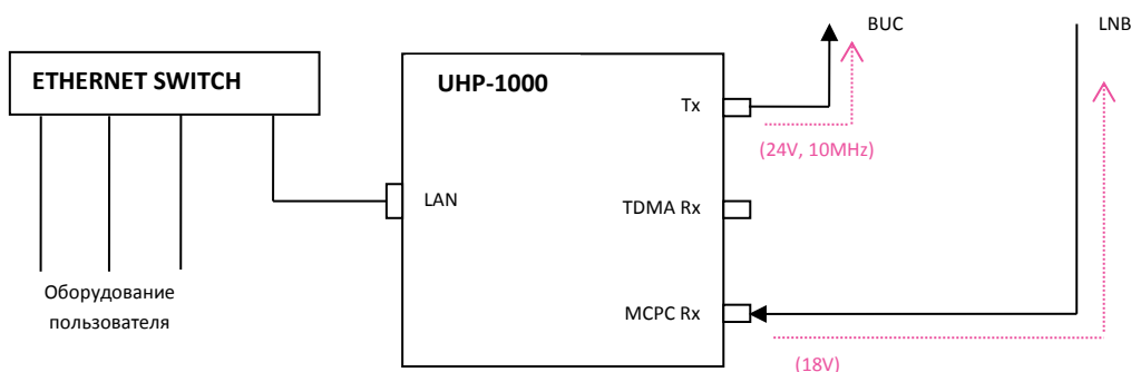
Рисунок 8 Пример подключения в режиме SCPC модема или TDM/TDMA терминала
