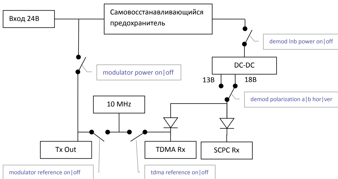
Рисунок 6 Управление питанием радиооборудования.
