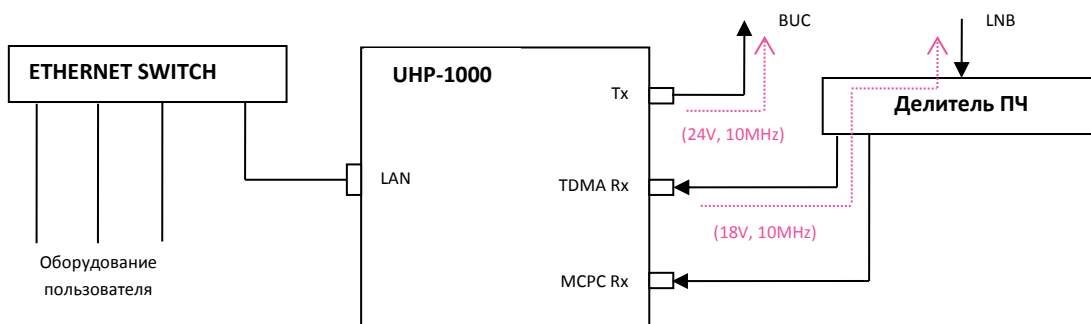
Рисунок 9 Пример подключения в режиме TDM/TDMA Mesh терминала
