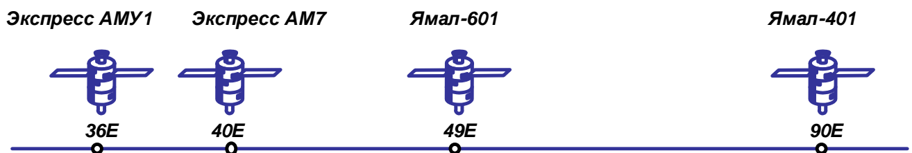
Рис. 2 Спутниковая группировка для оказания услуг связи
